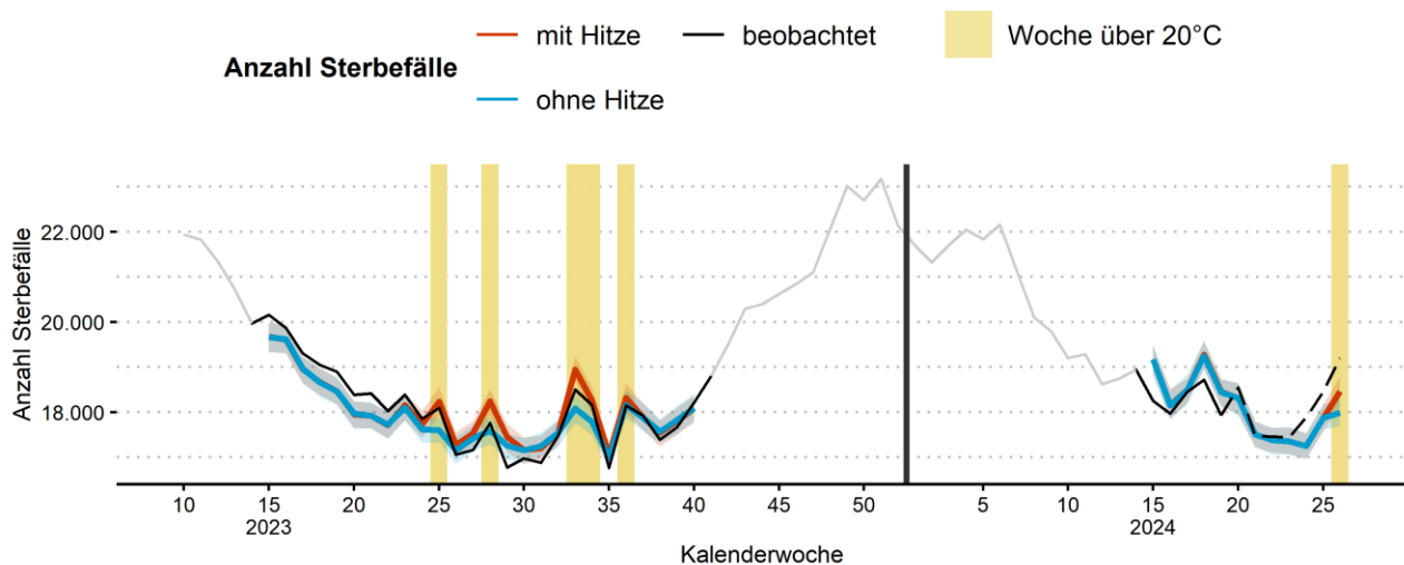
Abbildung 22. Verlauf der Sterbefallzahlen (schwarz) im Zeitraum 2023 bis KW 26/2024 wie vom Statistischen Bundesamt berichtet. Die Zahlen der letzten neun KW können noch durch Nachmeldungen beeinflusst werden und sind gestrichelt dargestellt. Außerhalb des Sommerhalbjahres (KW 15 bis 40) sind die Sterbefallzahlen ausgegraut. Die rote Linie zeigt den modellierten Verlauf der Anzahl von Sterbefällen mit Hitze, die blaue Linie den modellierten Verlauf ohne Hitze. Der Effekt der Hitze zeigt sich vor allem in Wochen, in denen die bundesweite Wochenmitteltemperatur 20°C überschreitet (gelbe Fläche). Wird die 20 °C Schwelle nur in einzelnen Bundesländern überschritten, können leichte Abweichungen zwischen der modellierten Anzahl von Sterbefällen mit und ohne Hitze (rote und blaue Linie) auch außerhalb gekennzeichnete Hitzewochen auftreten.
