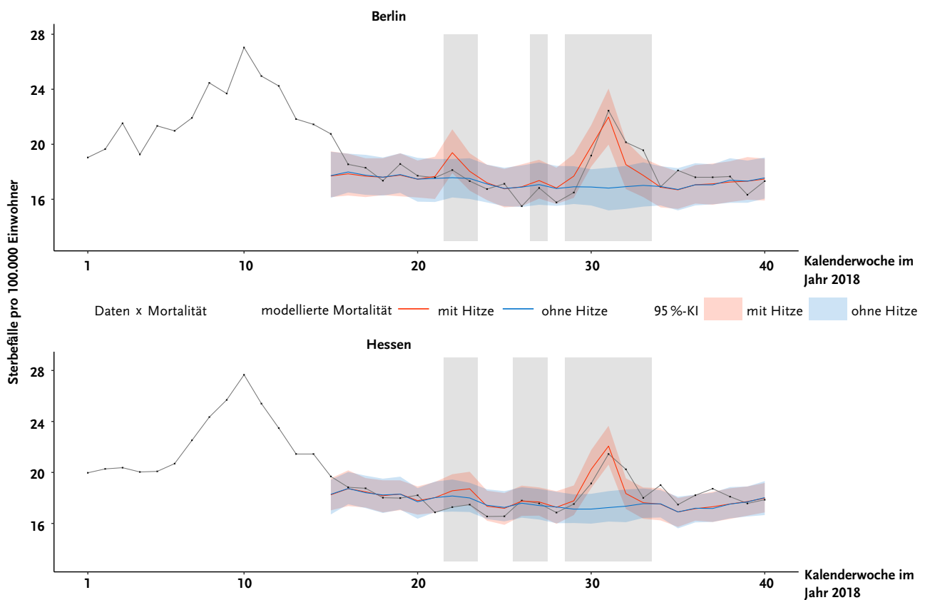
Abb. 3: Anpassung des generalisierten additiven Modells (GAM) an den Verlauf der Mortalität in Berlin und Hessen mit 95 %-Konfidenz-Intervall (95 %-KI) in den Kalenderwochen 1–40/2018, aggregiert über die Altersgruppen. Die vertikalen Bereiche in grau markieren Wochen mit Wochenmitteltemperatur über 20°C
