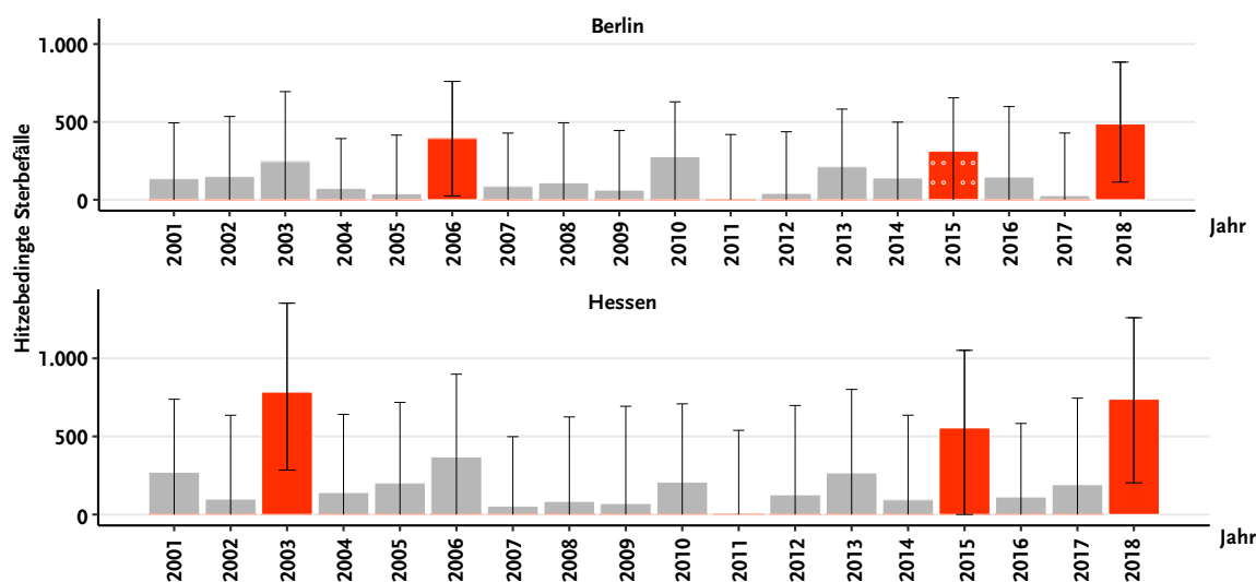
Abb. 5: Schätzung der hitzebedingten Sterbefälle in Berlin und Hessen zwischen 2001 und 2018 mit 95 %-Konfidenz-Intervall. Signifikant erhöhte Anzahlen sind in rot, grenzsignifikant erhöhte Anzahlen sind zusätzlich mit weißen Kreisen markiert
