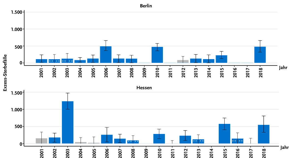
Abb. 6: Schätzung der Exzess-Mortalität in Berlin und Hessen zwischen 2001 und 2018 mit 95 %-Konfidenz-Intervall. Signifikant erhöhte Anzahlen sind in Blau, grenzsignifikant erhöhte Anzahlen sind zusätzlich mit weißen Kreisen markiert
