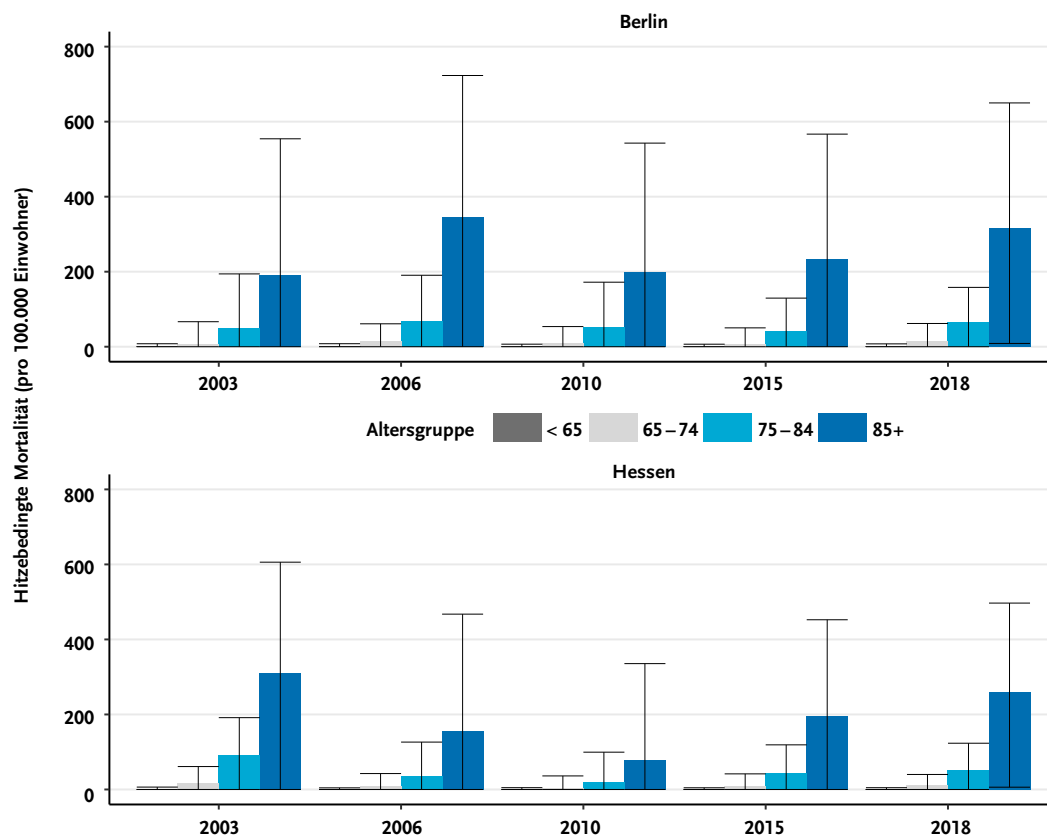
Abb. 9: Schätzung der hitzebedingten Mortalitätsrate in Berlin und Hessen zwischen 2001 und 2018 mit 95 %-Konfidenz-Intervall
