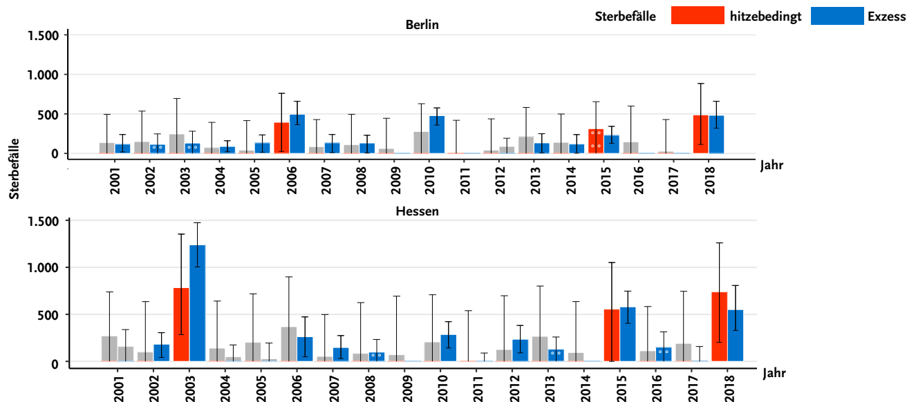
Abb. 7: Vergleich der Schätzung der hitzebedingten Sterbefälle und der Exzess-Mortalität in den Jahren 2001–2018 in Berlin und Hessen mit 95 %-Konfidenz-Intervallen, signifikant erhöhte Anzahlen sind Rot bzw. Blau, grenzsignifikant erhöhte sind zusätzlich mit weißen Kreisen markiert
