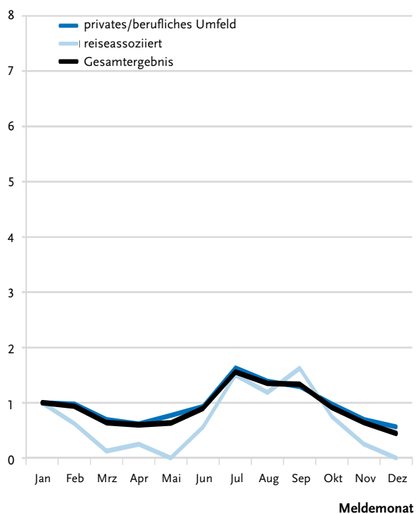
Abb. 7 | Fälle von Legionärskrankheit nach Meldemonat und Expositions-kategorie, Deutschland 2019 (N=1.548 Fälle) im Vergleich zu 2020 (N=1.281 Fälle). Darstellung linke Seite: absolute Fallzahlen (A/C); Darstellung rechte Seite: Fallzahlen relativ zum Monat Januar als Referenz (B/D). Relative Fallzahlen in (B) und (D): Expositions-kategorie Krankenhaus, Pflegeeinrichtung und sonstiger Expositions-ort nicht dargestellt.
