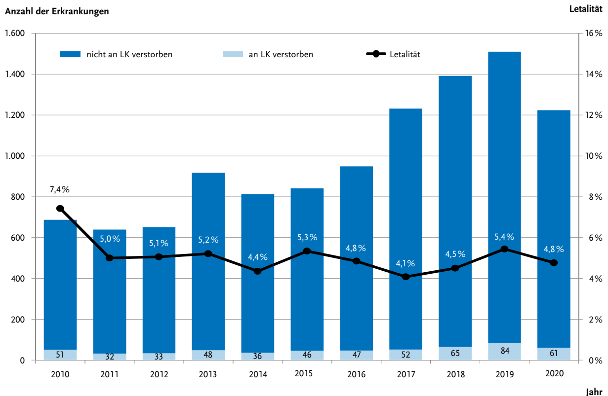
Abb. 8 | Anzahl der an das RKI übermittelten Erkrankungen und Todesfälle von Legionärskrankheit (LK) sowie die Letalität, Deutschland, 2010–2020.
