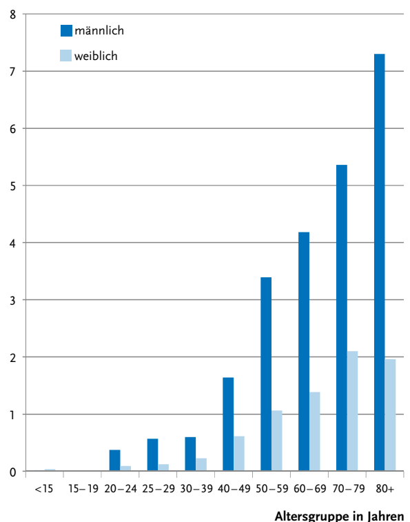
Abb. 3 | An das RKI übermittelte Fälle von Legionärskrankheit pro 100.000 Einwohner nach Altersgruppe und Geschlecht, Deutschland, 2020 (N=1.278).
